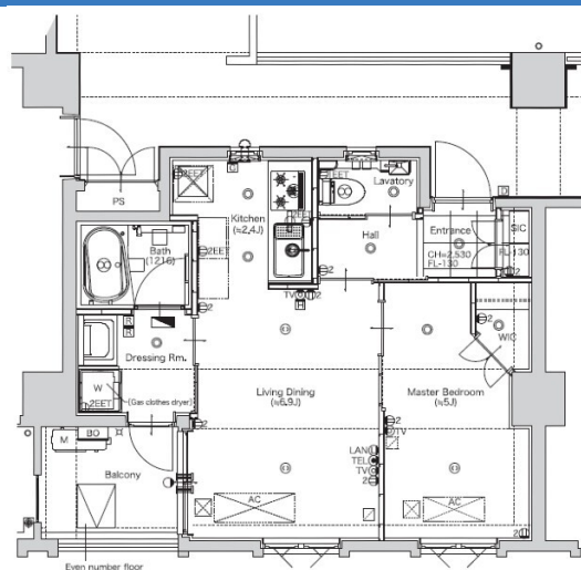
物件間取
